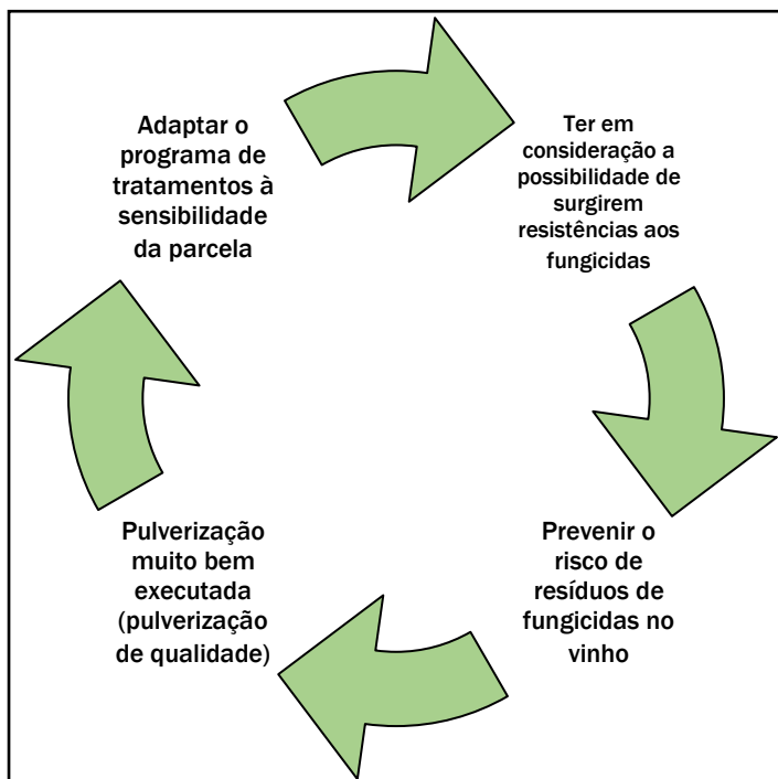
Figura 1. Condições para o êxito da proteção contra a Botrytis na Vinha (adaptado de N. Muckensturm & M. Decoin, Phytoma, 525, mars 2000, 50-52 )
